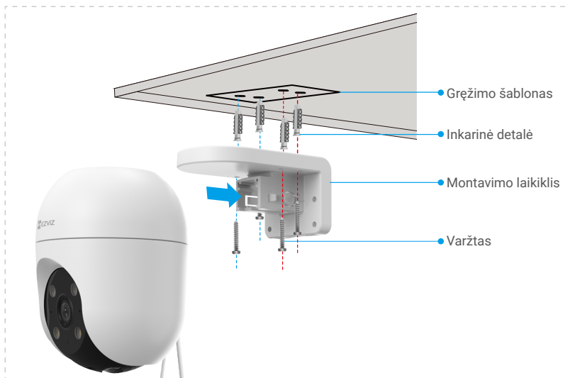
1 pav. Lubinis laikiklis
