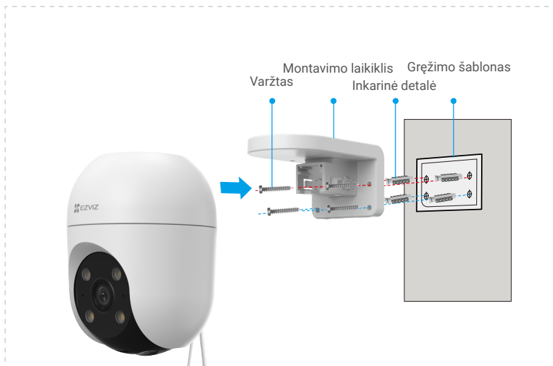
2 pav. Sieninis laikiklis
